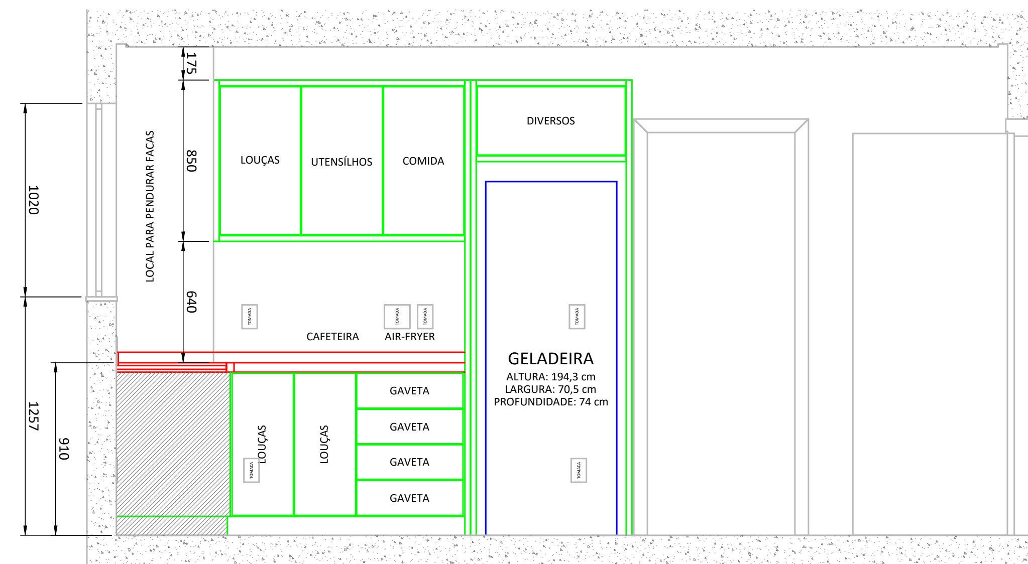
CORTE BB
